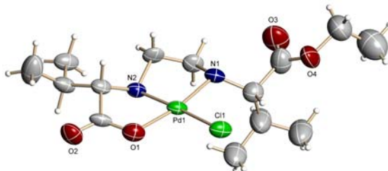
Slika 1. Struktura dobijenog kompleksa
