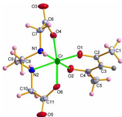
Fig. 1: s-cis -[Cr(edda)(acac)]
