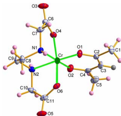
Slika 1. s-cis -[Cr(edda)(acac)]
