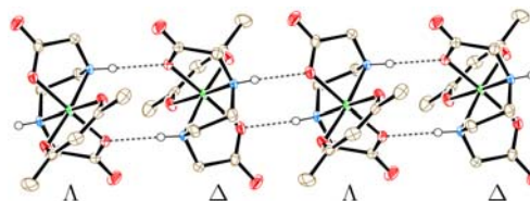
Slika 2. Vodonične veze u s-cis -[Cr(edda)(acac)]
