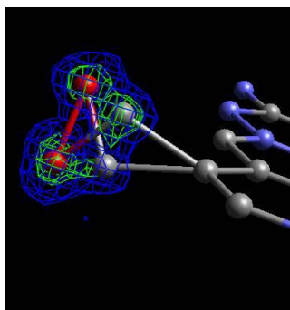
Slika 1. Trodimenzionalna slika koje pokazuje razliku u elektronskoj gustini i neuredjenost -CH 2 OH grupe
