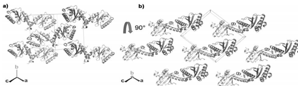
Kristalno pakovanje MjRelB – MjRelE proteinskog kompleksa u dve projekcije
