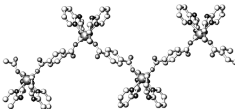
Slika 2. Prikaz cik-cak lanca posmatrano približno duž a -ose ( c -osa je horizontalna).
