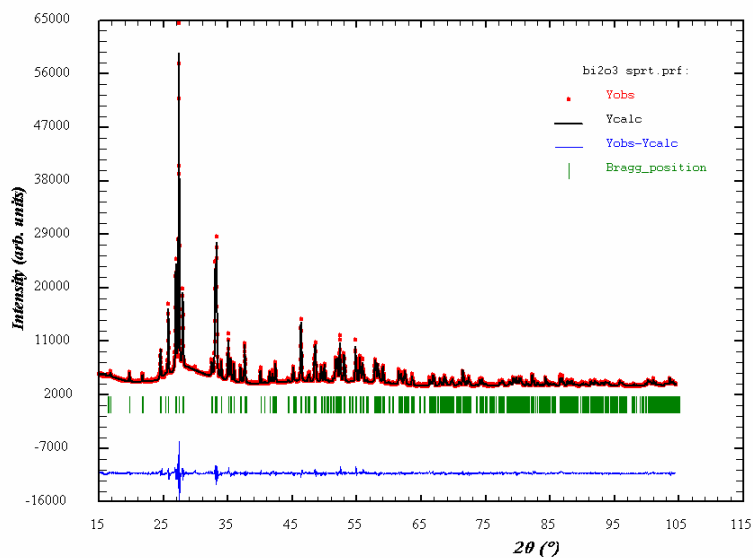
Slika 1. Dijagram praha nakon Ritveldovog utičnjavanja
